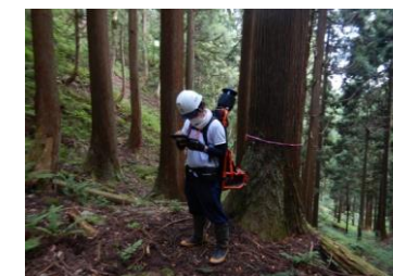
林内測量機器による測量の様子
