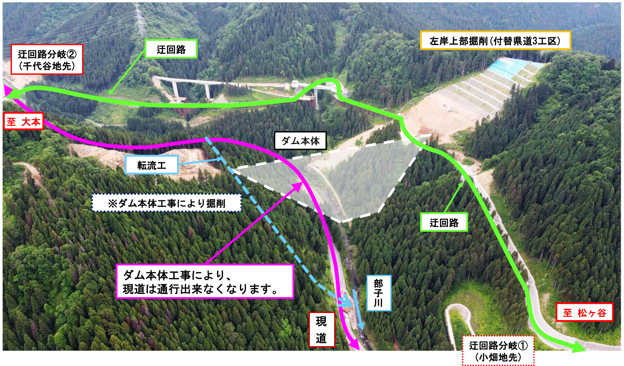
迂回路: 全景 (小畑地区側より撮影)
